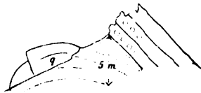
Fig. 5. Biegungen im Glimmerquarzit am Contact beim Gasteinhorn
